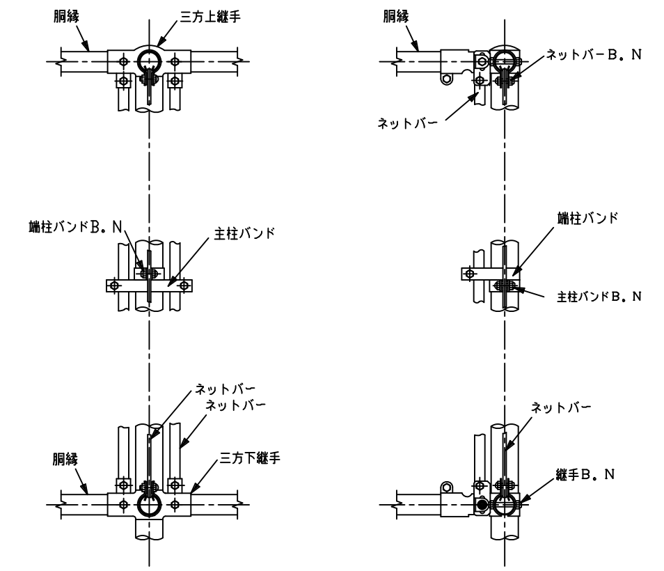
三方部取付詳細
