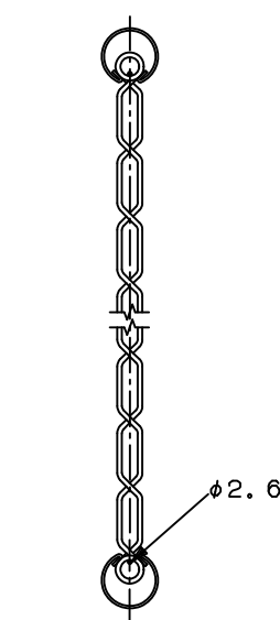
胴縁と金網取付断面図
