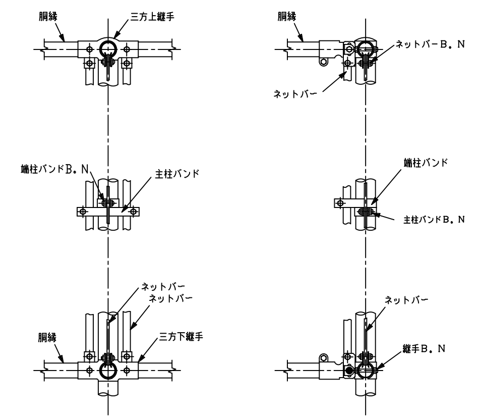
三方部取付詳細
