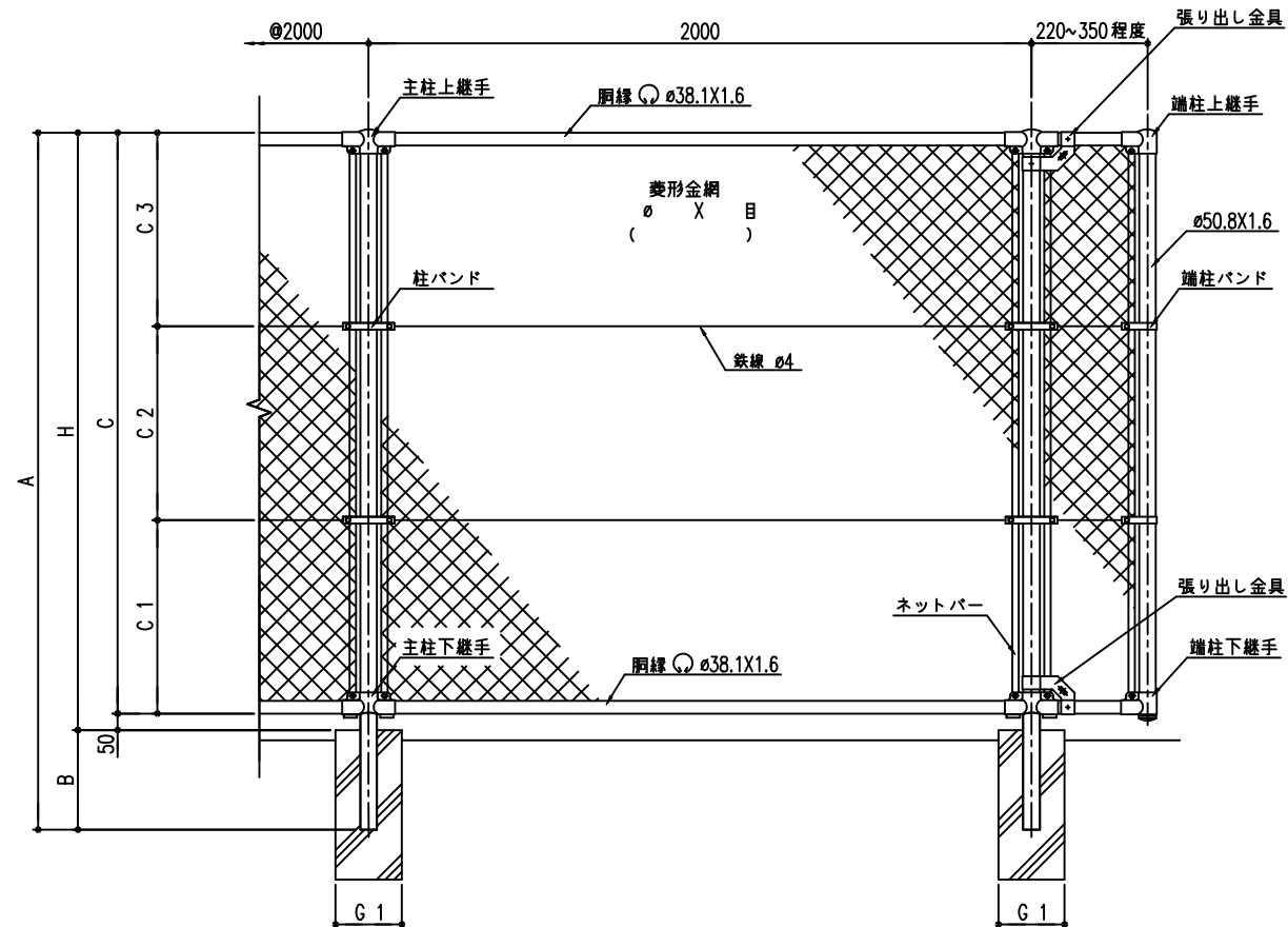
正面図 S=1/15
