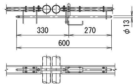
カンヌキ取付詳細図
