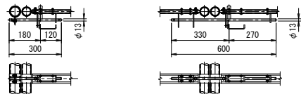
カンヌキ取付詳細図
