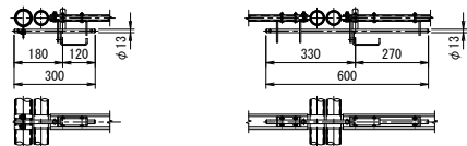
カンスキ取付詳細図
