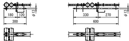
カンスキ取付詳細図
