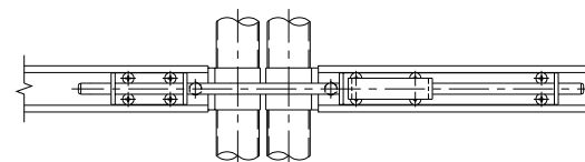
カヌキ取付詳細図
