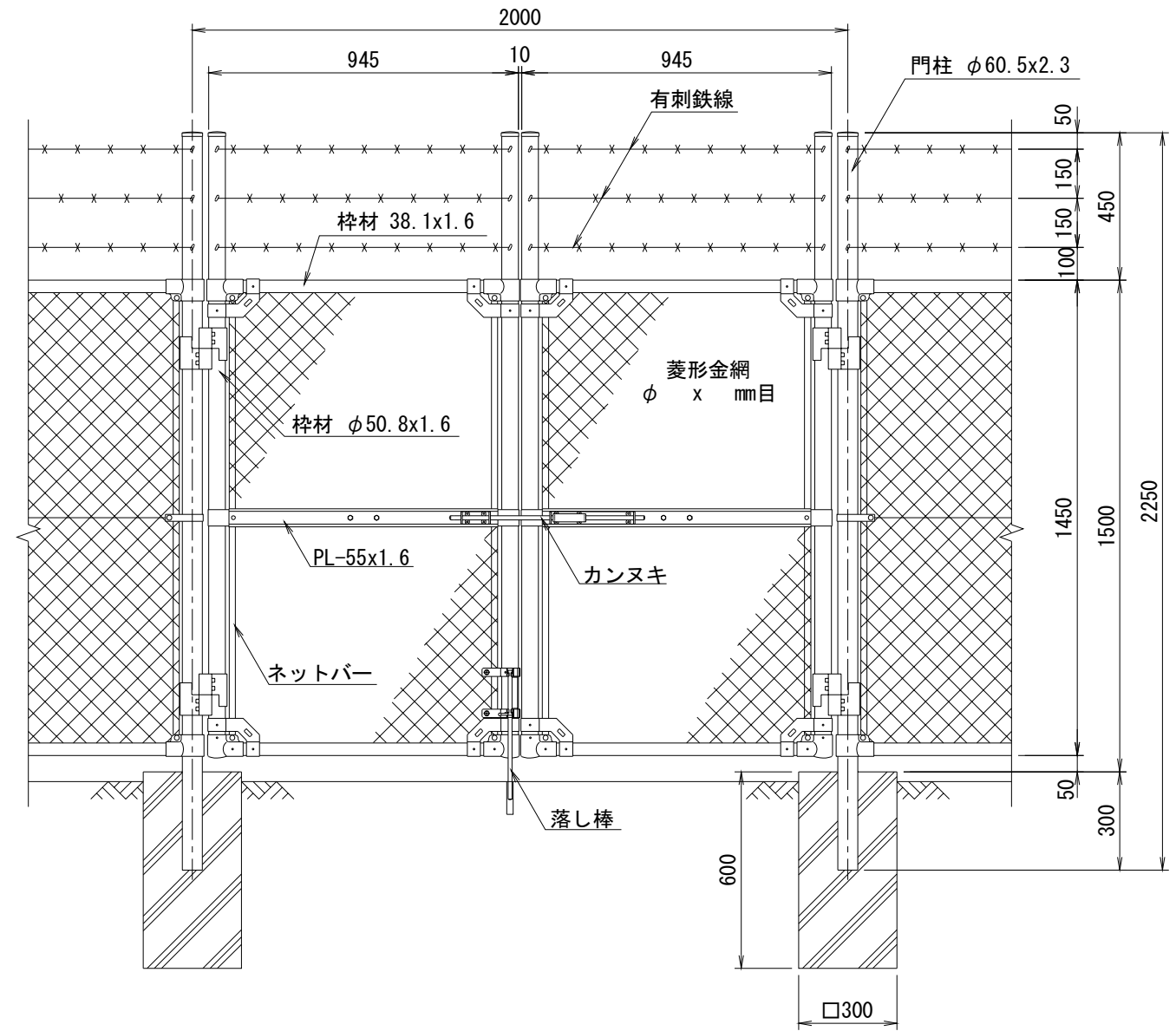
正面図 (S=1/20)
