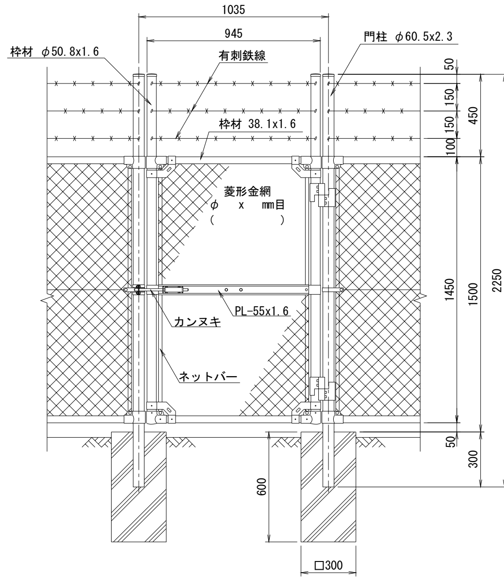
正面図 (S=1/20)
