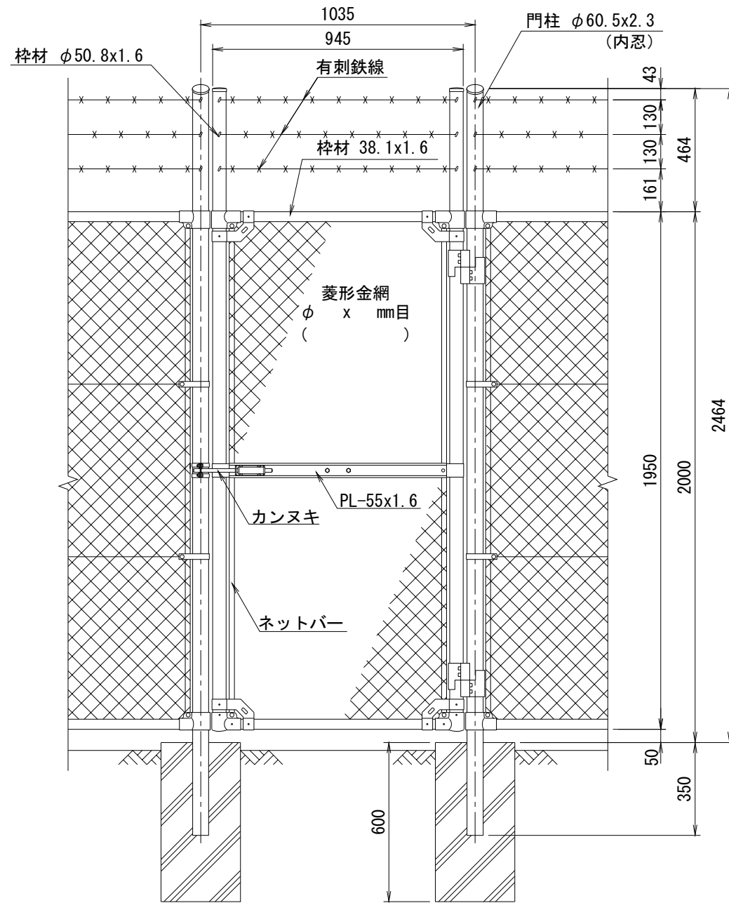
正面図 (S=1/20)
