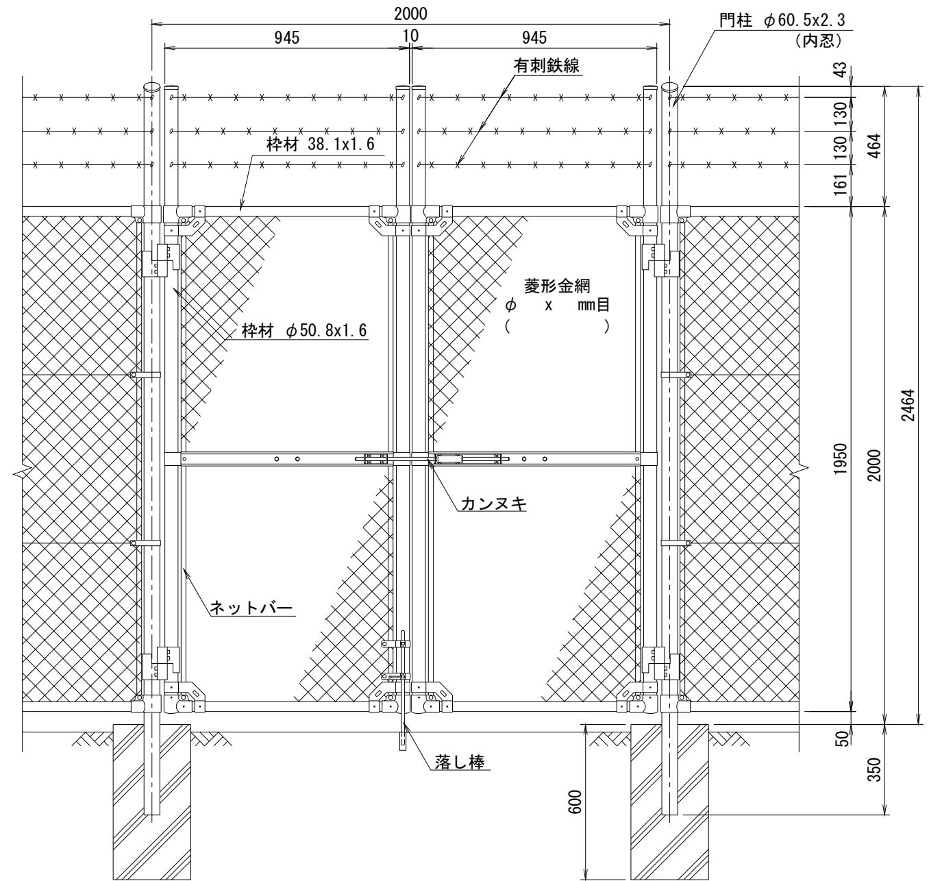
正面図 (S=1/20)
