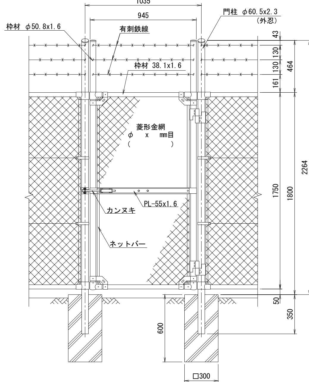
正面図
