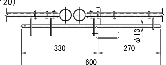
正面図
