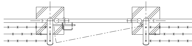
平面図
