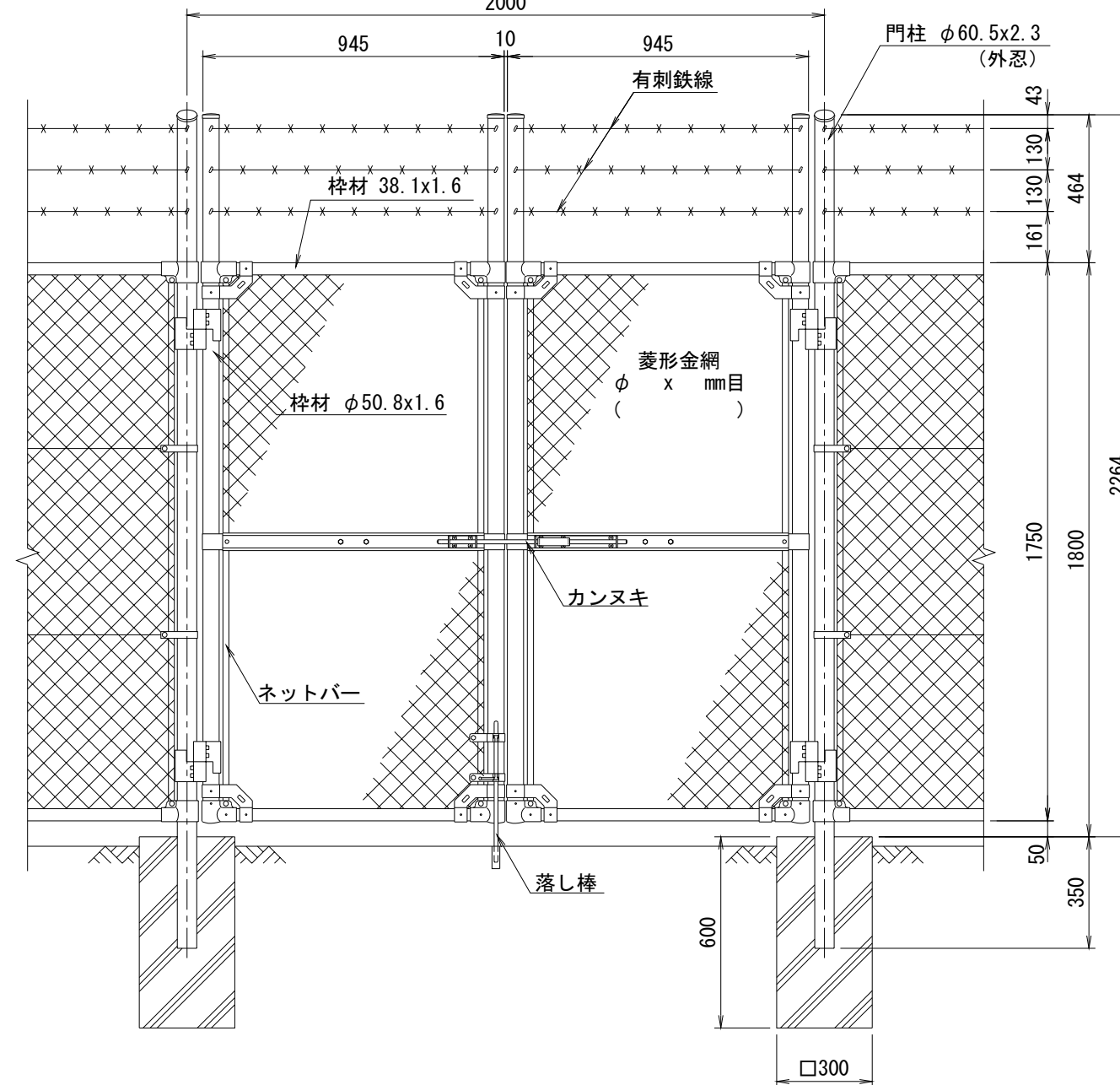
正面図
