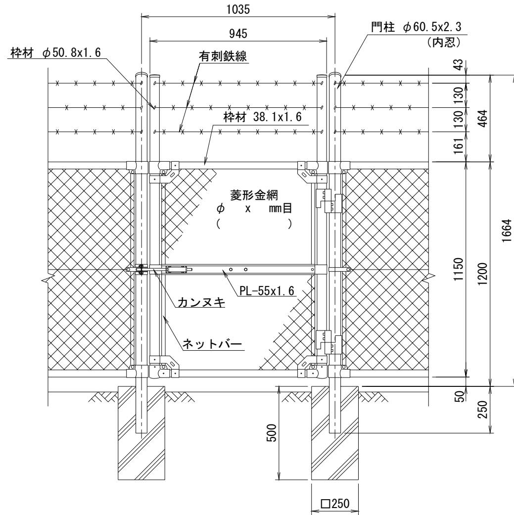
正面図 (S=1/20)
