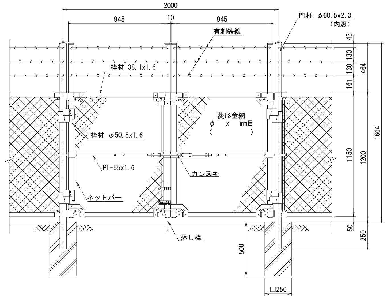
正面図 (S=1/20)
