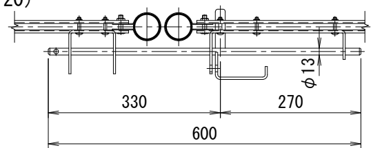
正面図 (S=1/20)
