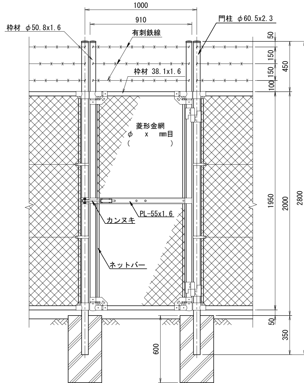
正面図 (S=1/20)
