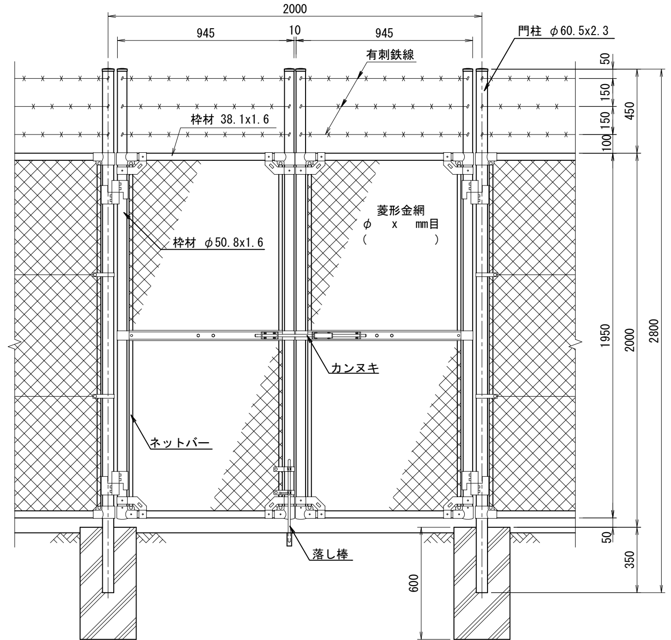
正面図 (S=1/20)
