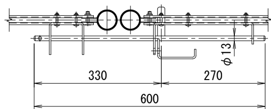
正面図 (S=1/20)
