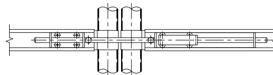
カンヌキ取付詳細図
