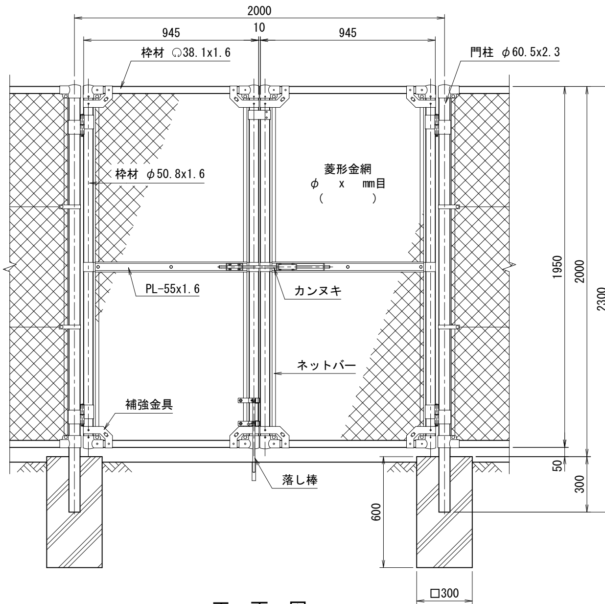
正面図 (S=1/20)
