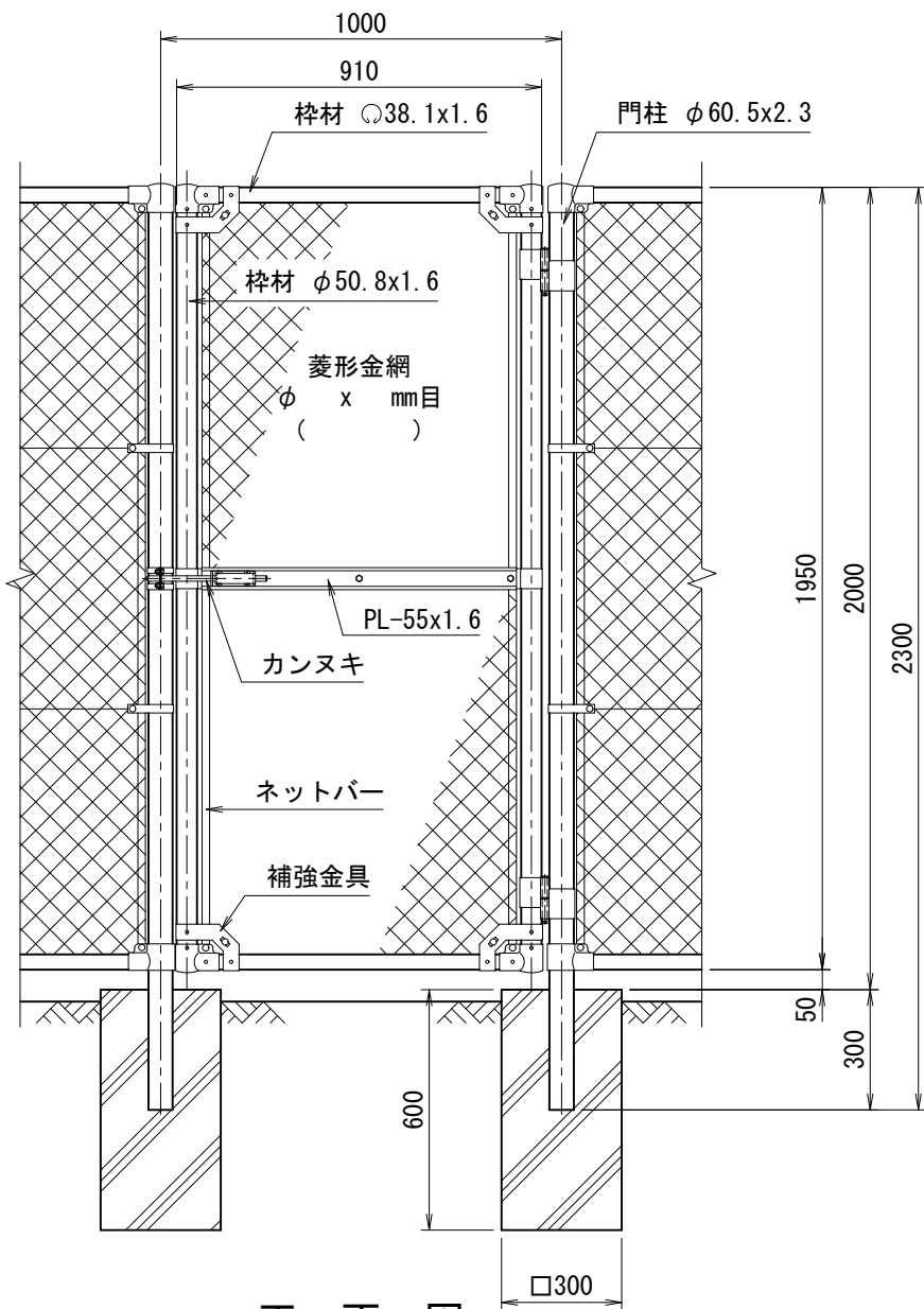
正面図 (S=1/20)
