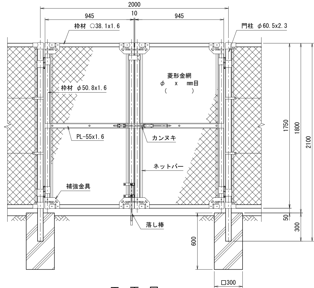
正面図 (S=1/20)
