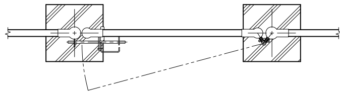
平面図 (S=1/20)
