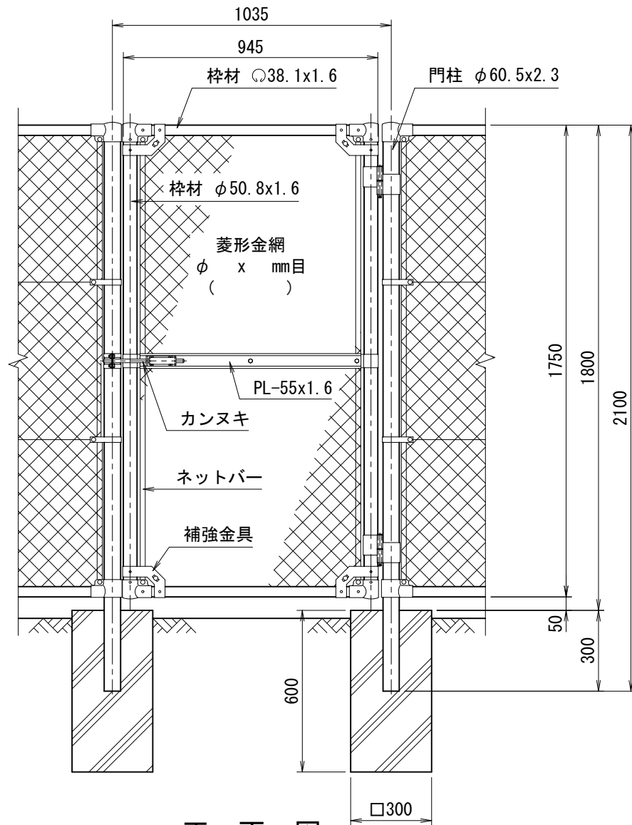
正面図 (S=1/20)
