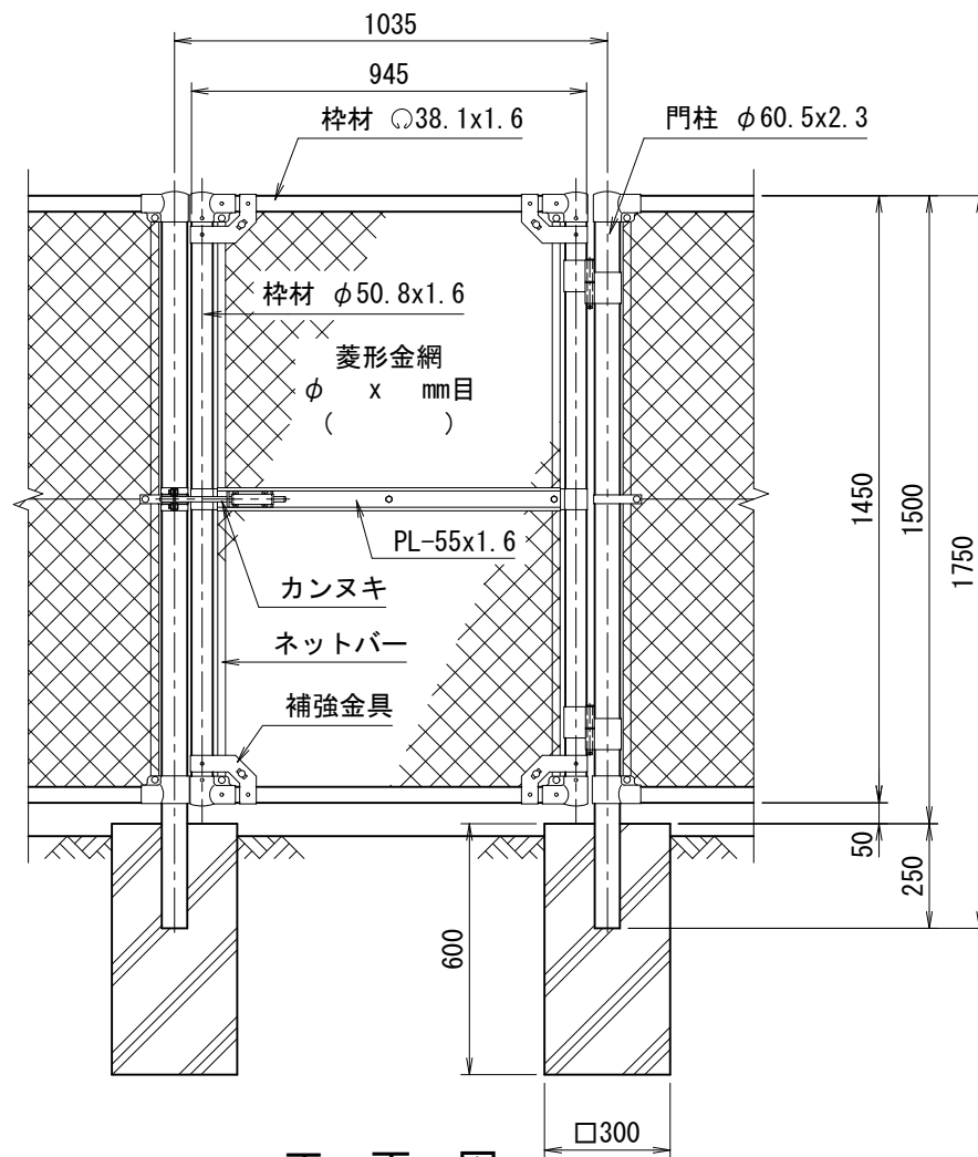
正面図 (S=1/20)
