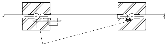
平面図 (S=1/20)
