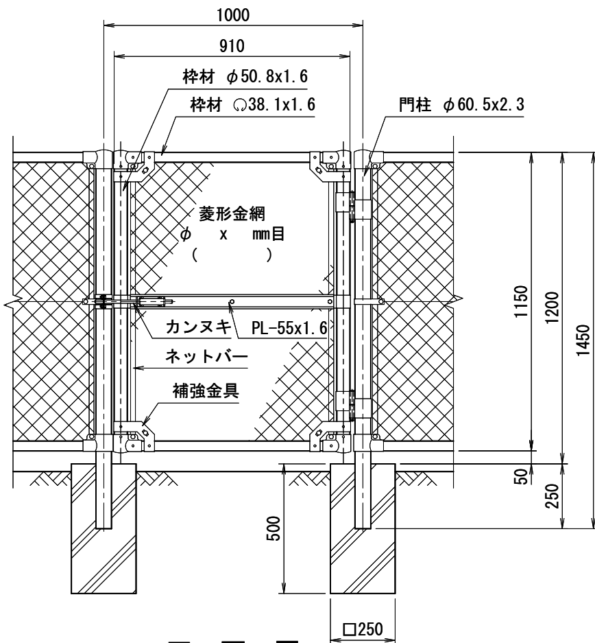
正面図 (S=1/20)
