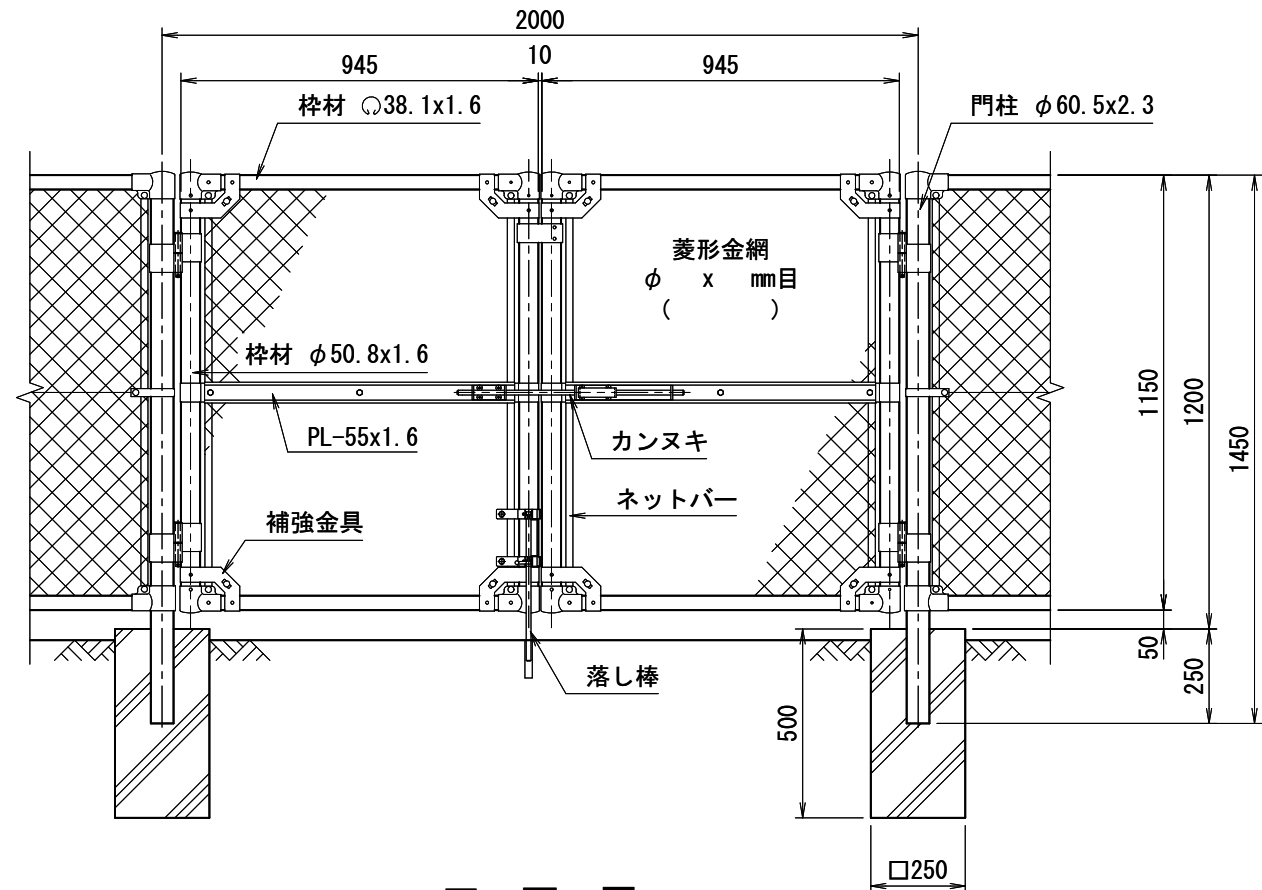
正面図 (S=1/20)
