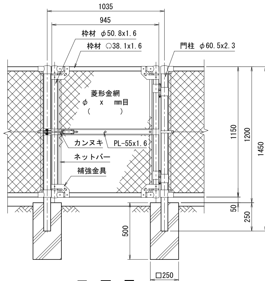
正面図 (S=1/20)
