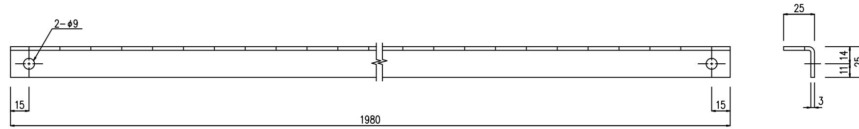
平面図 S=1/2
