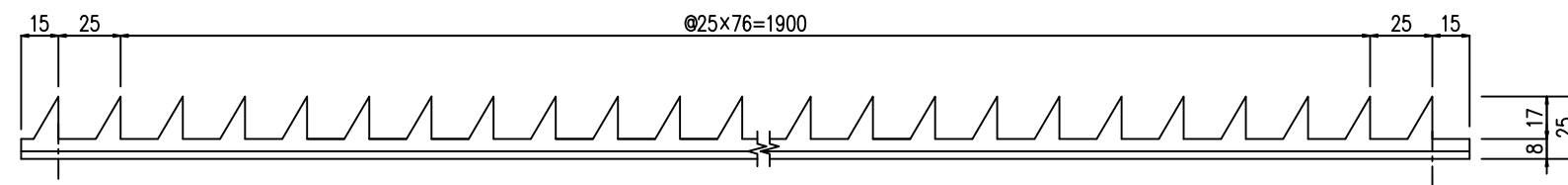
正面図 S=1/2
