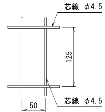
パネル詳細図
