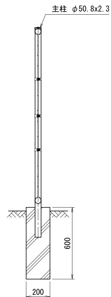
側面図 (S=1/20)
