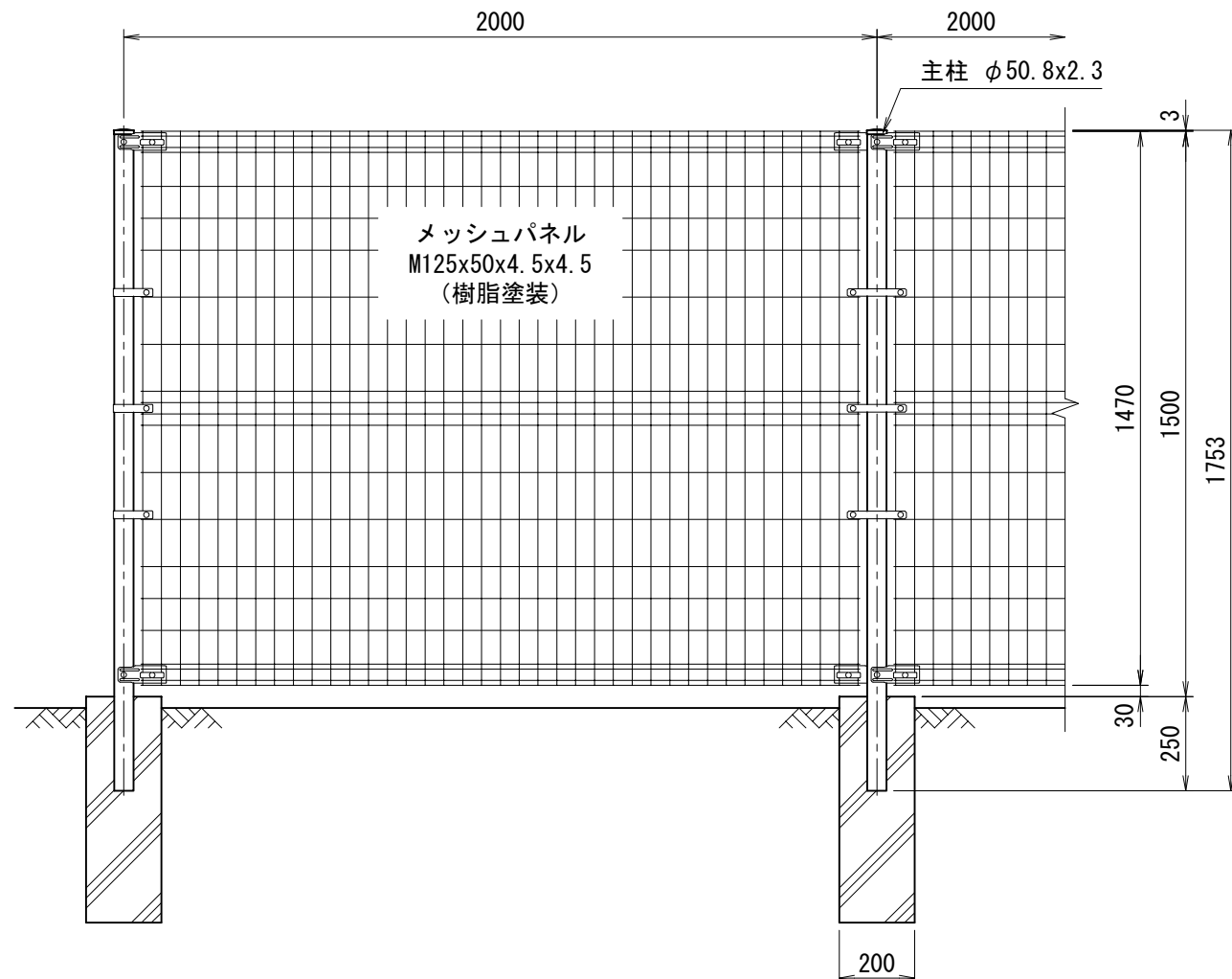
正面図 (S=1/20)
