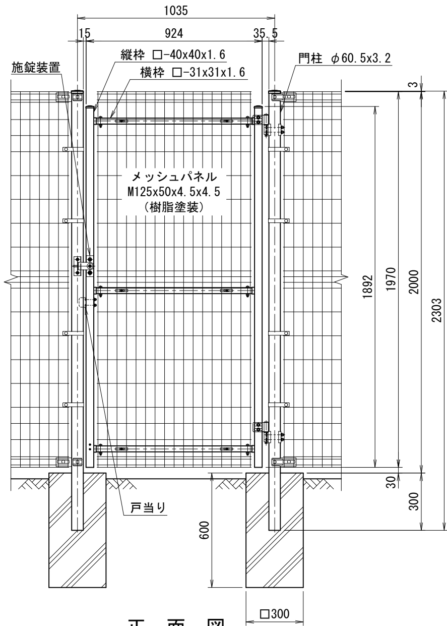
正面図 (S=1/20)
