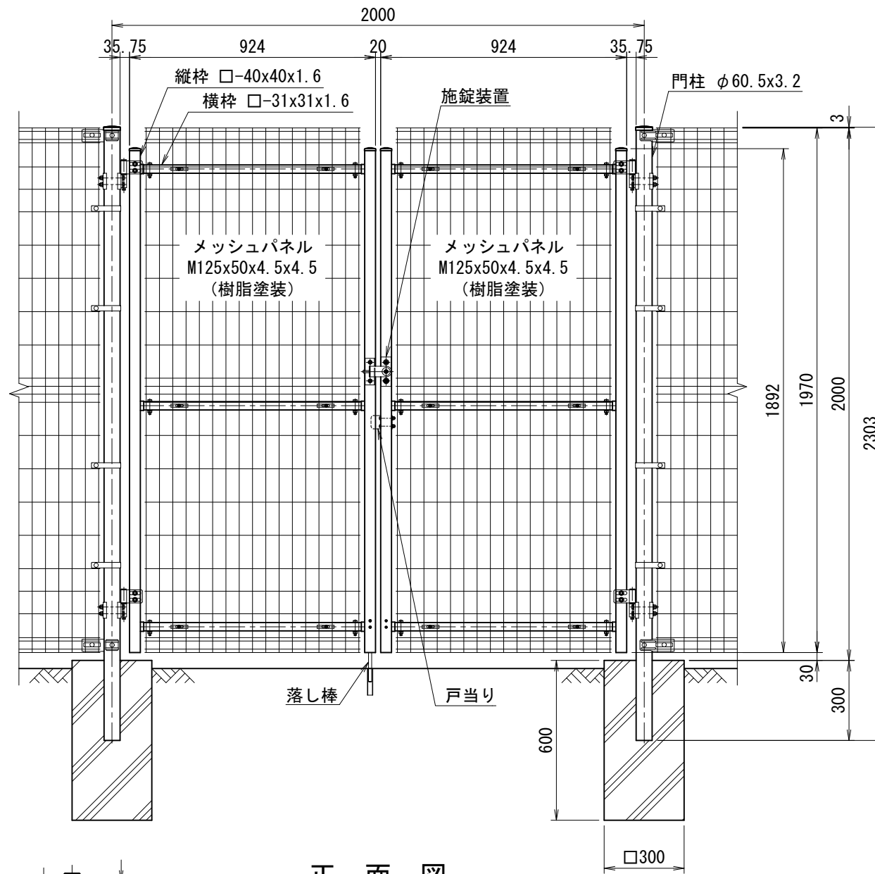
正面図 (S=1/20)
