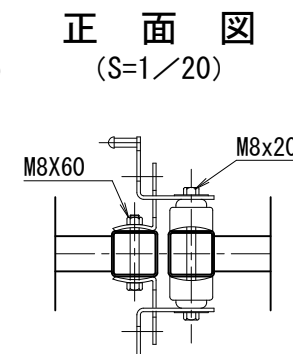
両開き施錠詳細図
