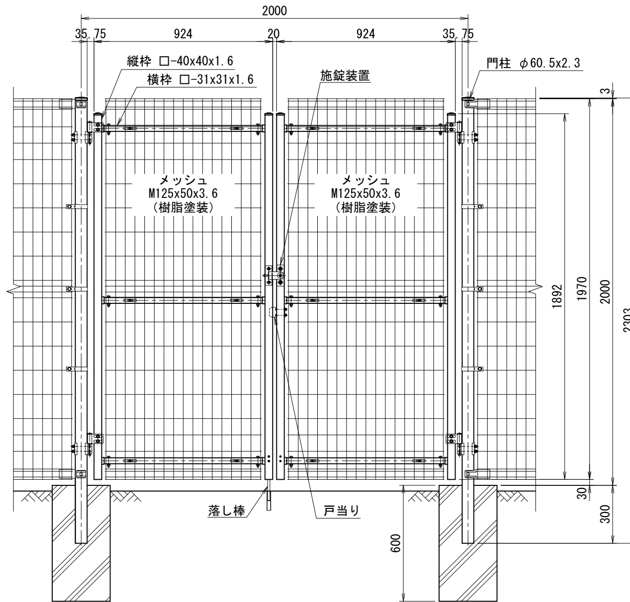
正面図 (S=1/20)
