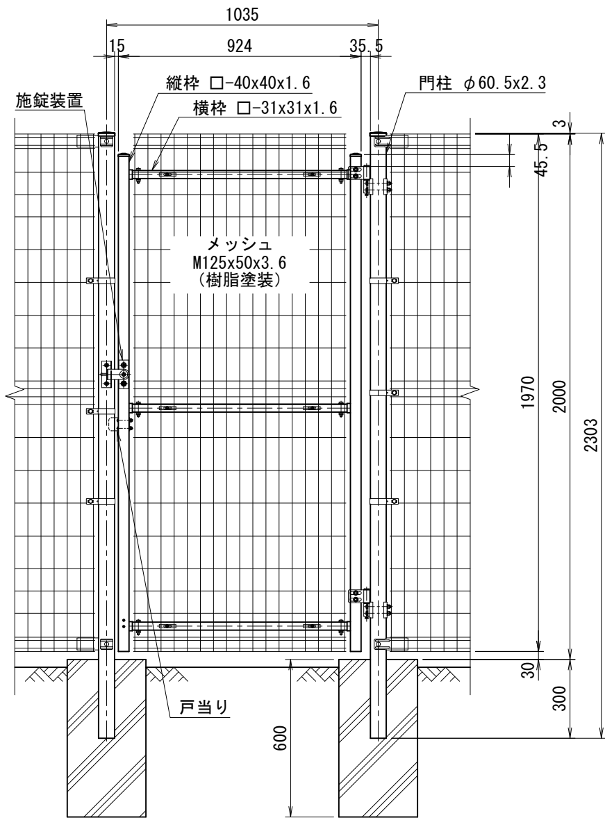
正面図 (S=1/20)
