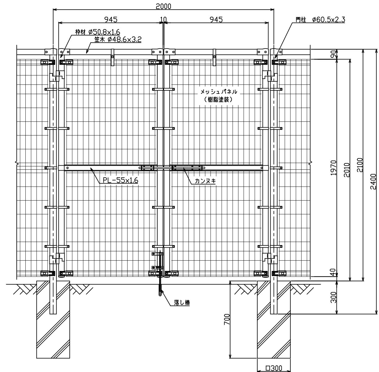
正面図 S=1/15
