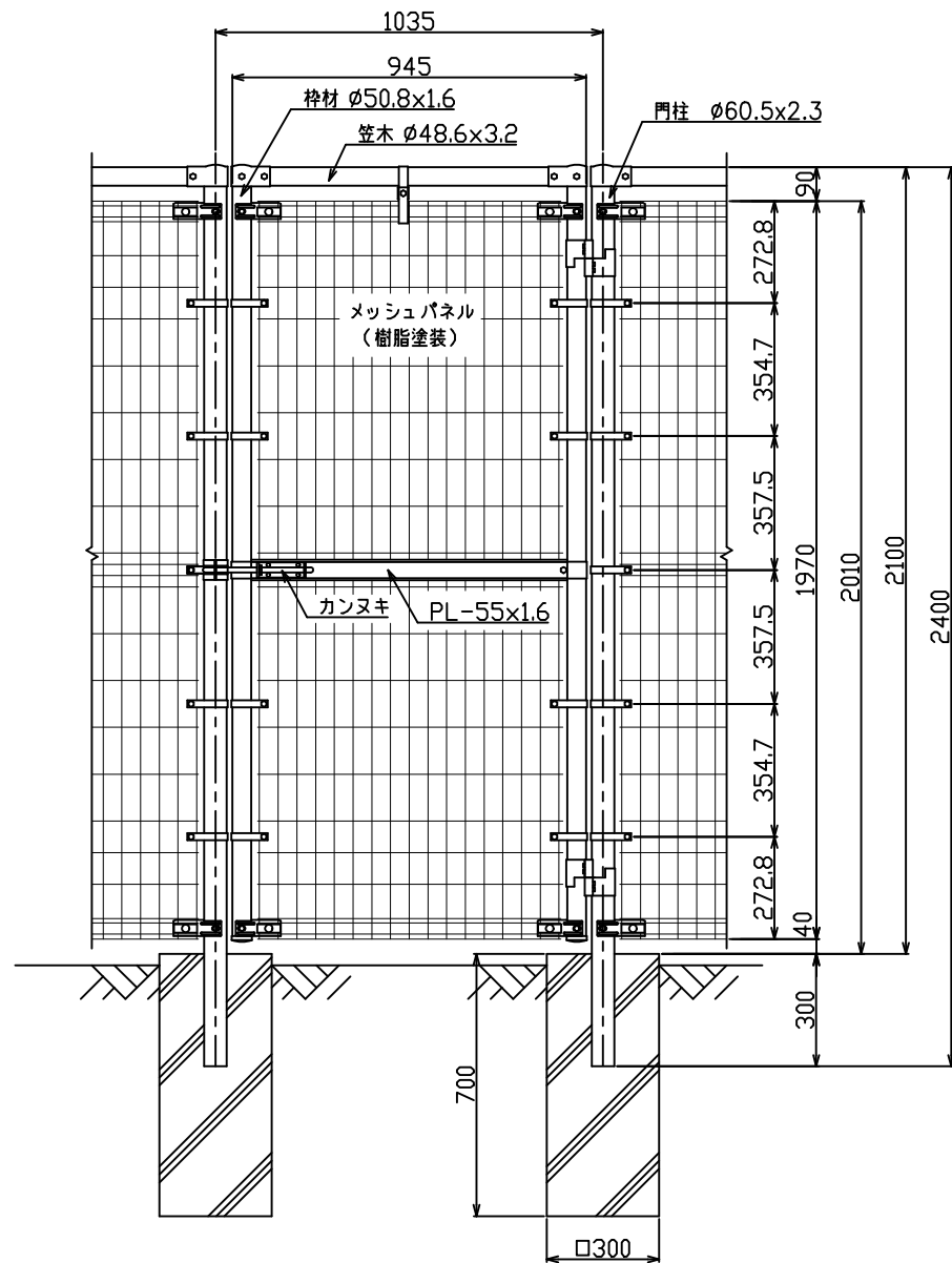
正面図 S=1/15
