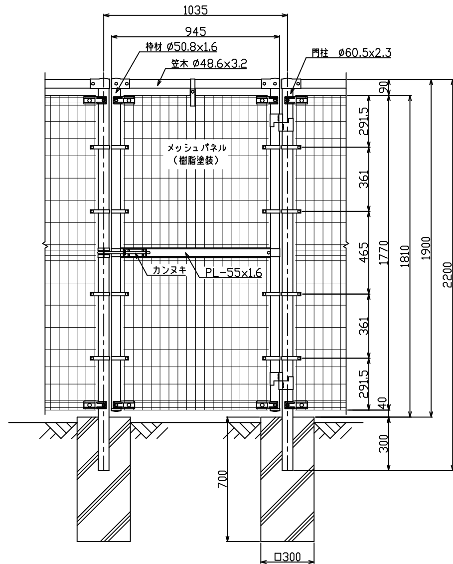
正面図 S=1/15
