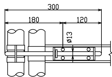
片開カンヌキ詳細図 S=1/5
