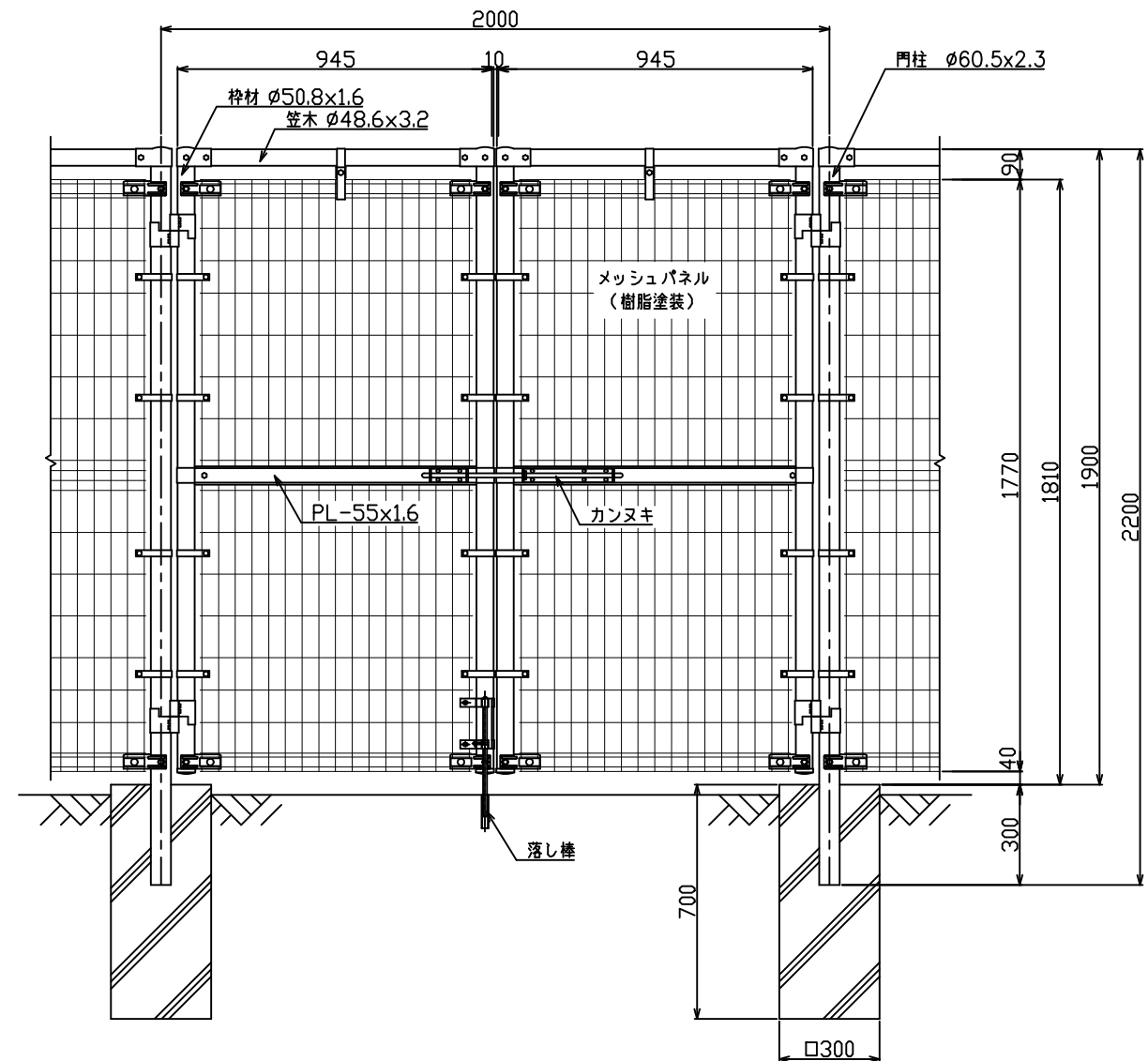
正面図 S=1/15
