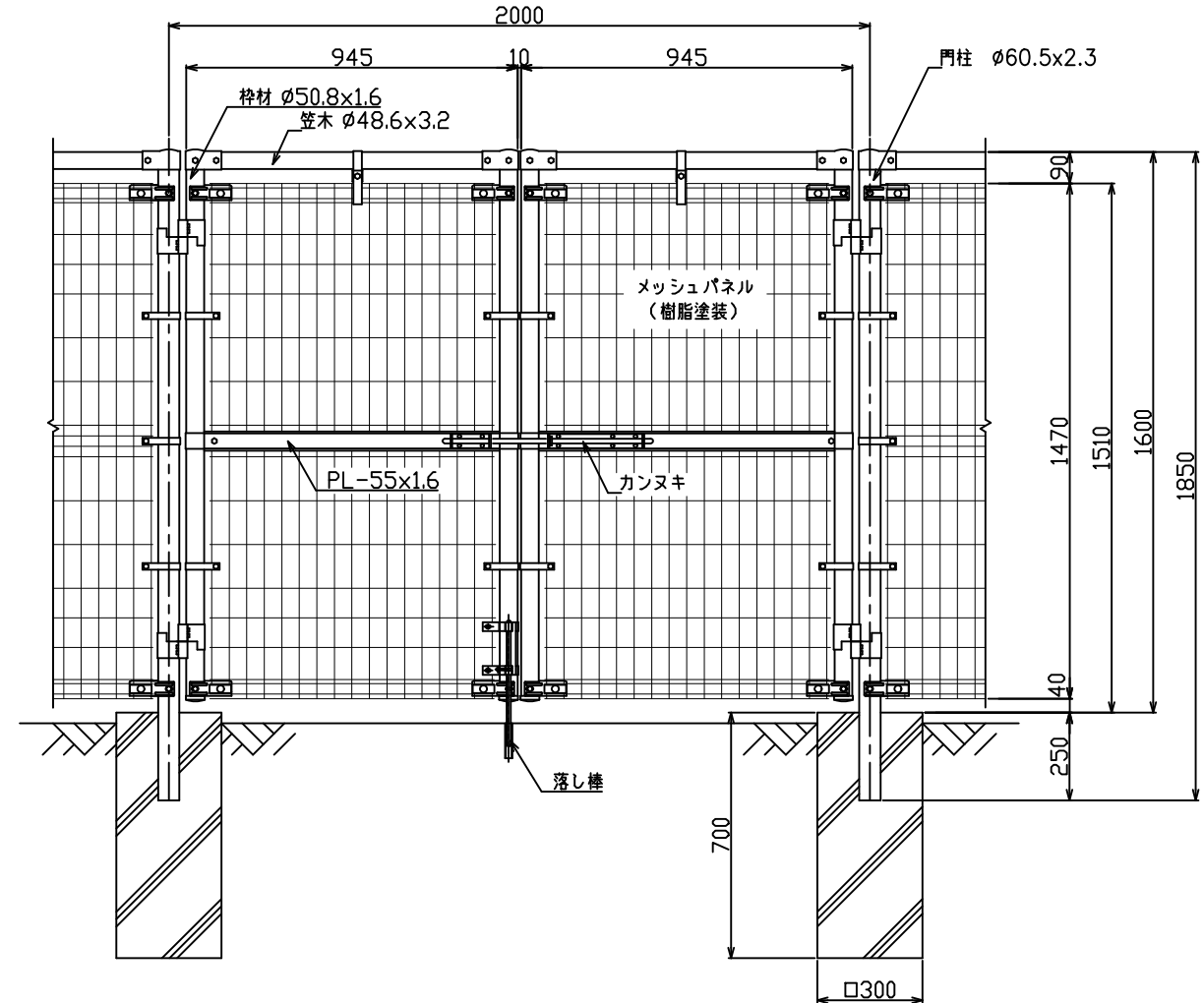
正面図 S=1/15
