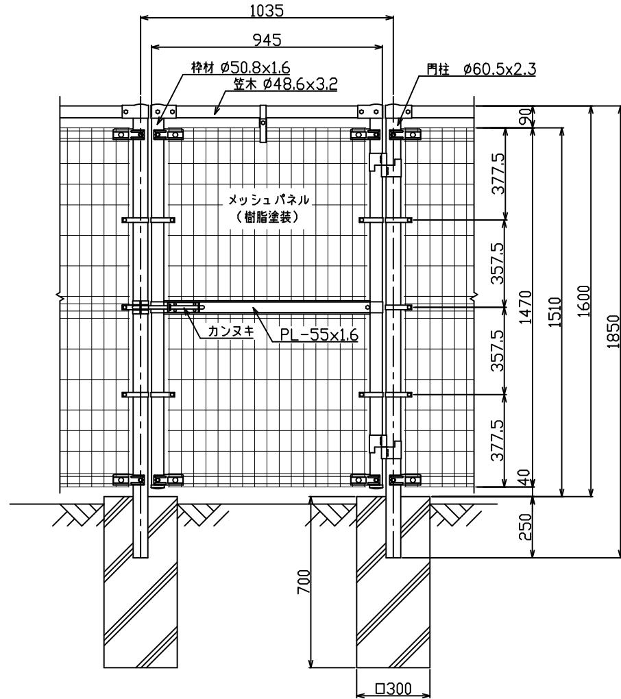
正面図 S=1/15
