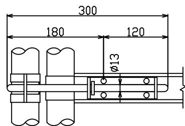
片開カヌキ詳細図 S=1/5
