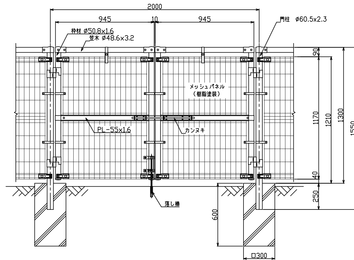
正面図 S=1/15
