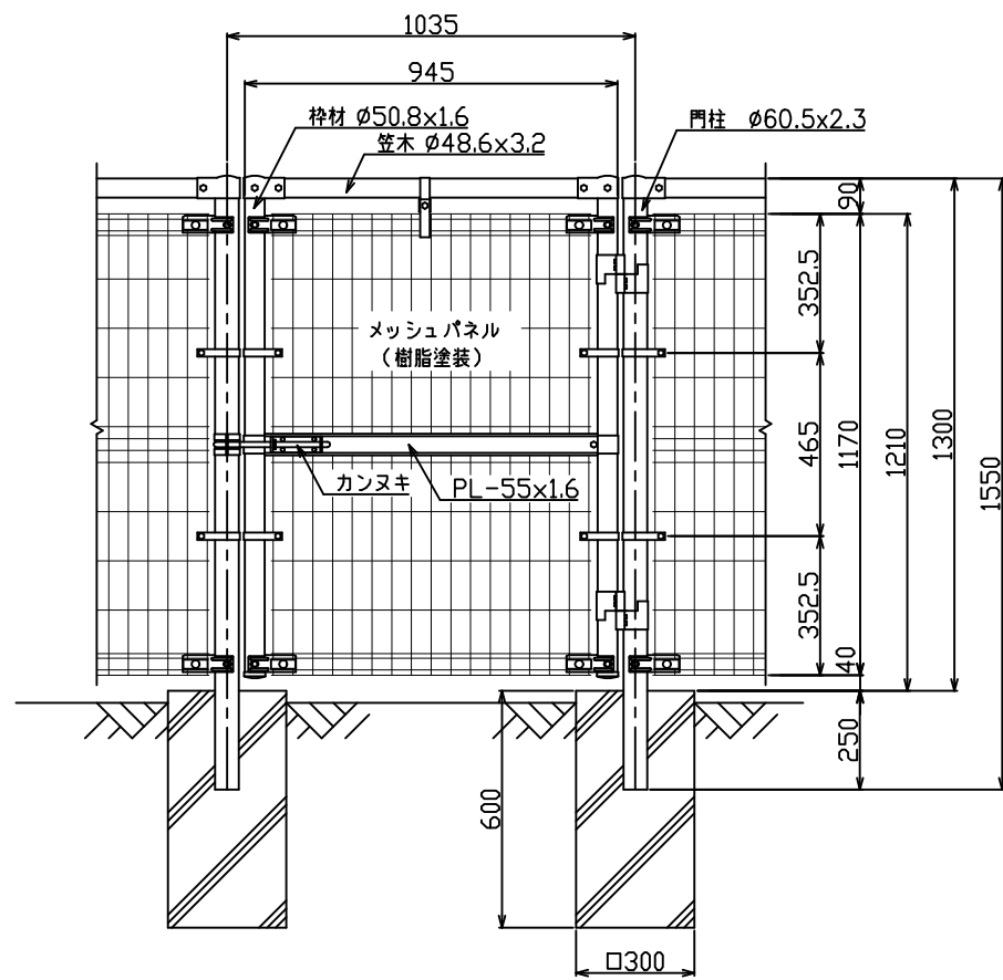
正面図 S=1/15
