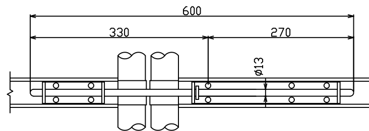
両開カヌキ詳細図 S=1/5
