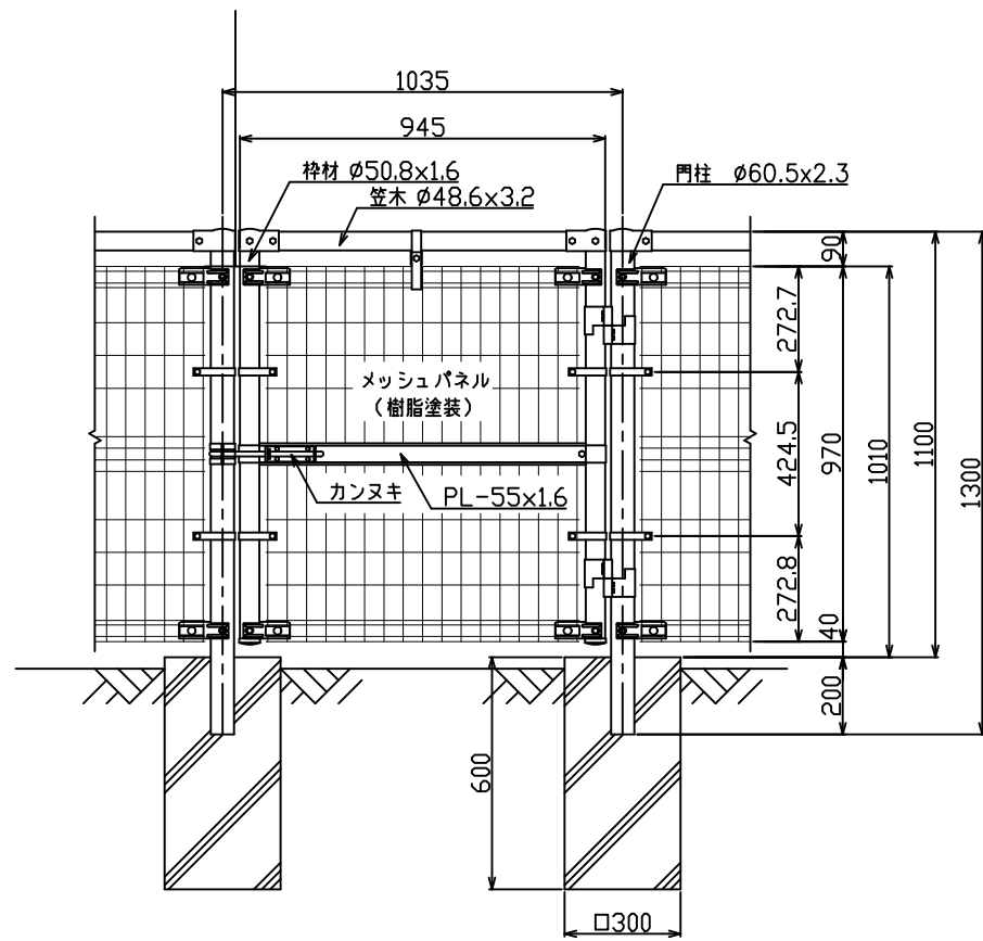
正面図 S=1/15
