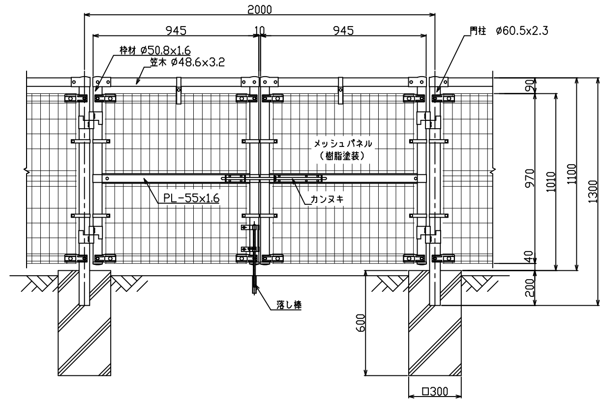
正面図 S=1/15
