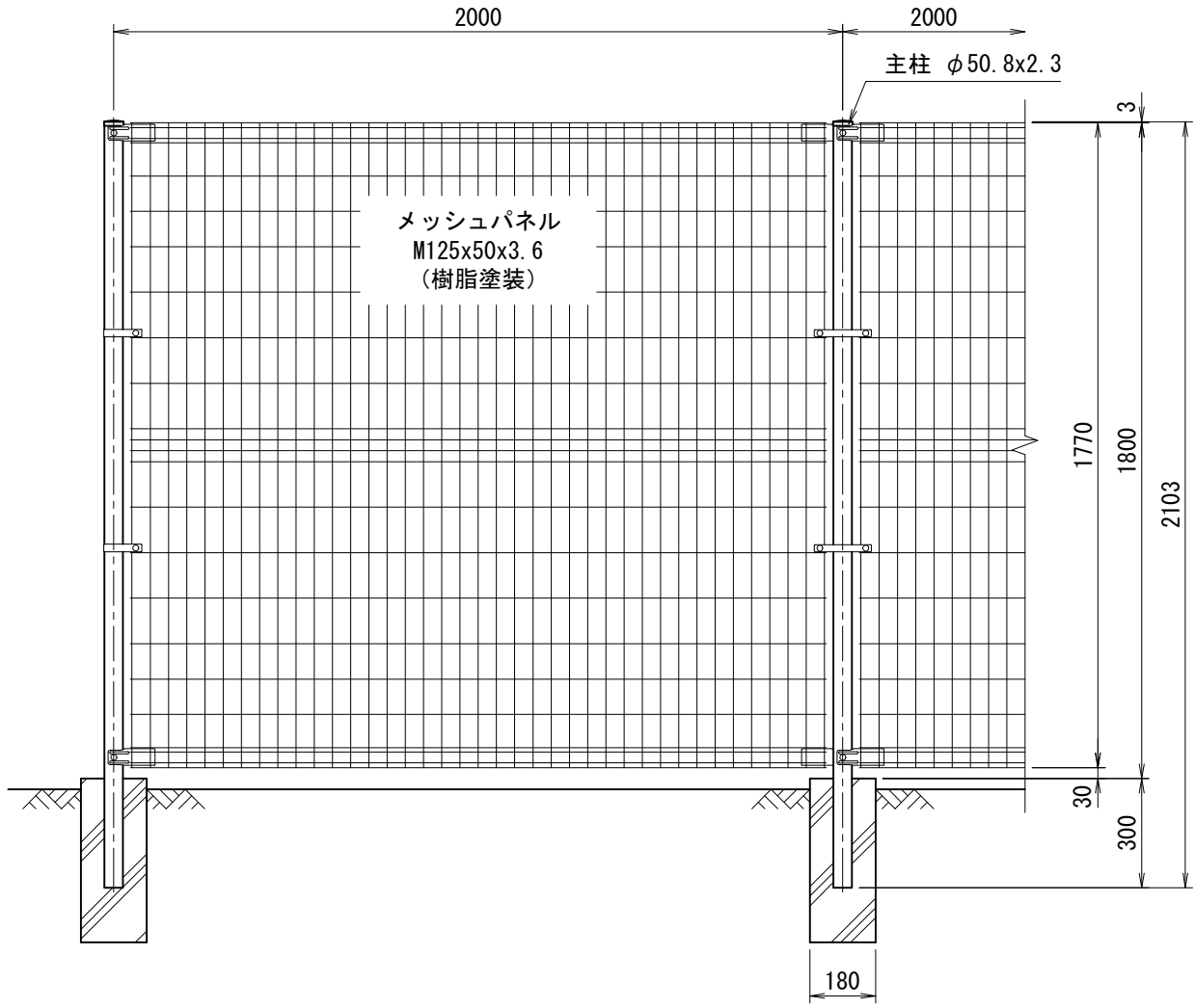
正面図 (S=1/20)
