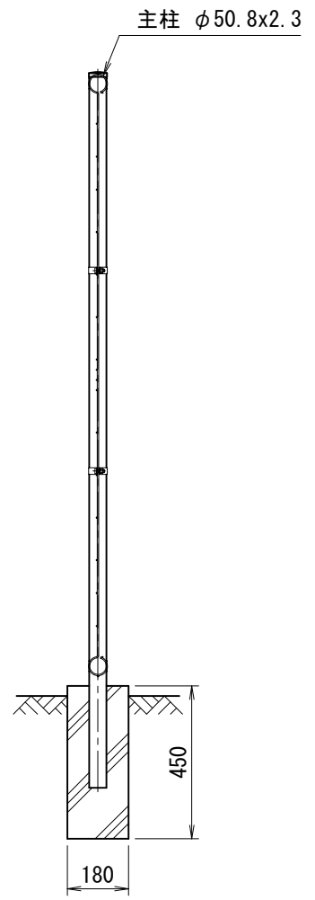
側面図 (S=1/20)
