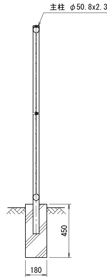
側面図 (S=1/20)
