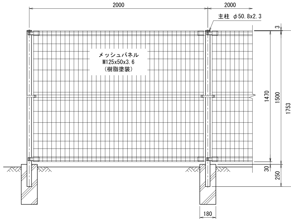
正面図 (S=1/20)
