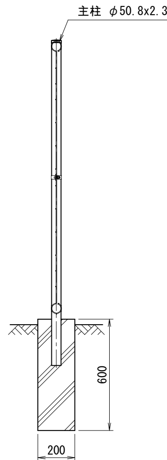
側面図 (S=1/20)
