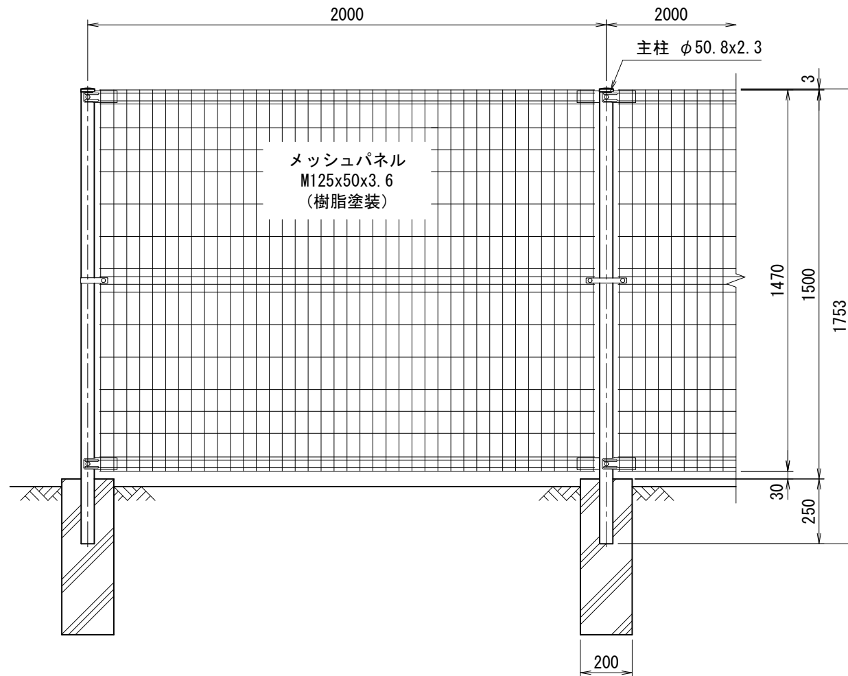
正面図 (S=1/20)
