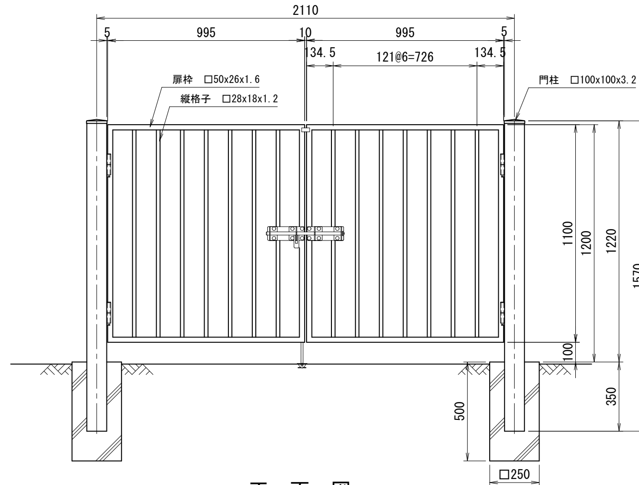
正面図 (S=1/20)
