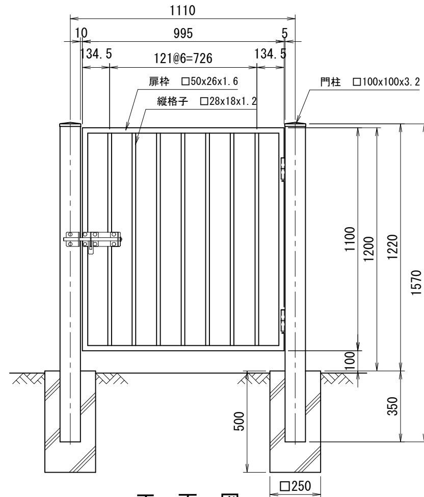
正面図 (S=1/20)
