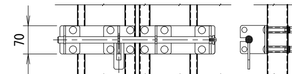
カンヌキ取付詳細図
