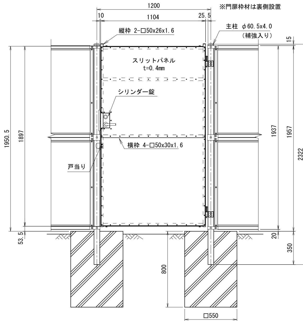
正面図 (S=1/20)
