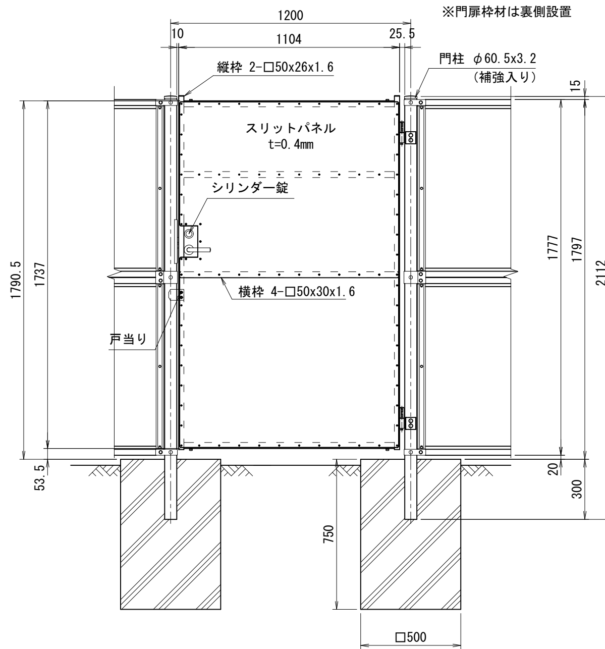
正面図 (S=1/20)
