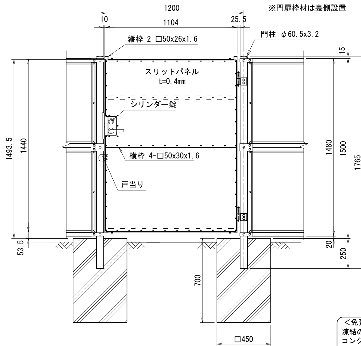
正面図 (S=1/20)
