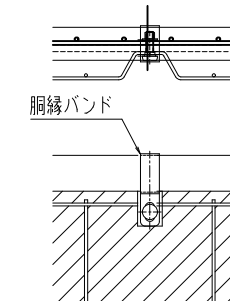
胴縁バンド部 S=1/10
