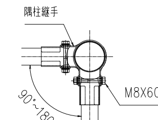
コーナー部 S=1/10
