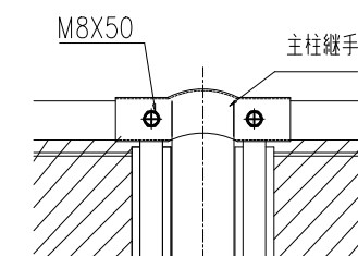
支柱継手部 S=1/10
