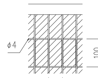
背面メッシュ部 S=1/10
