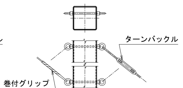
中ブレース取付詳細
