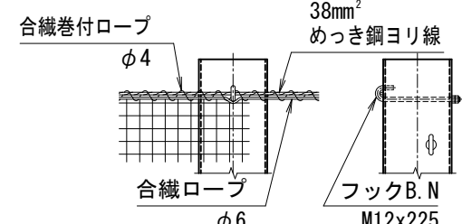
主柱・ワイヤー取付詳細
