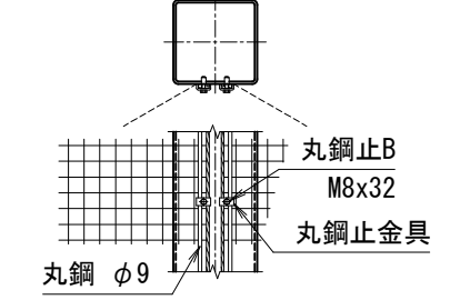
隅柱・ネット取付詳細
