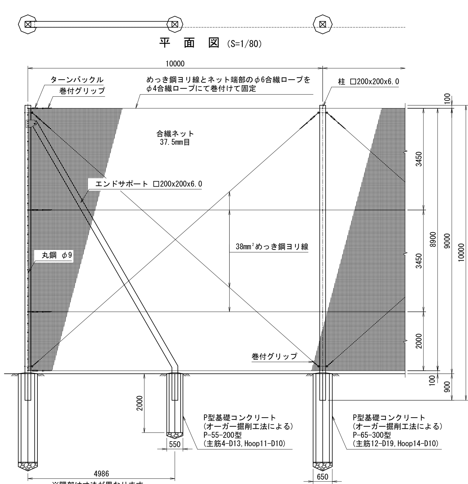
正面図 (S=1/80)
