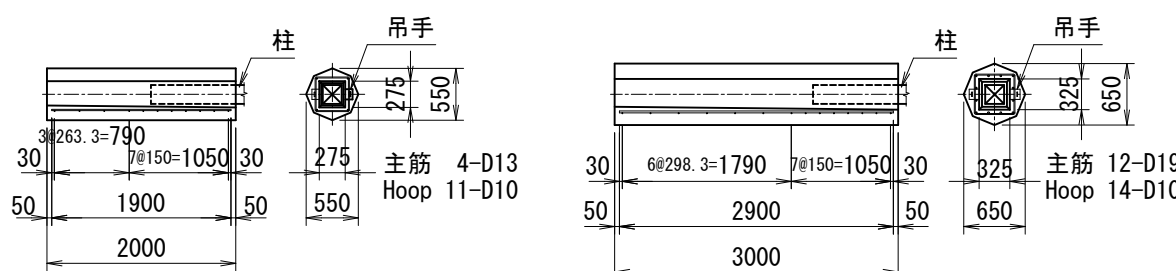
P型基礎コンクリート配筋図
