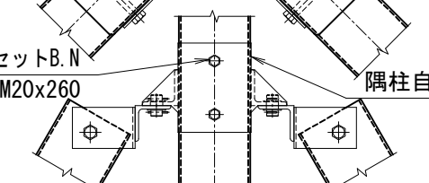
隅柱・ワイヤー取付詳細
