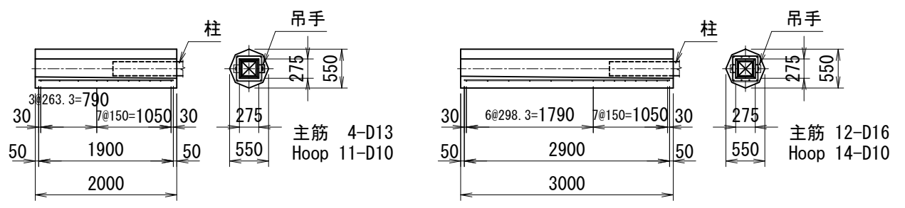
P型基礎コンクリート配筋図
