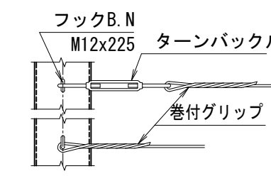
端柱・ワイヤー取付詳細
