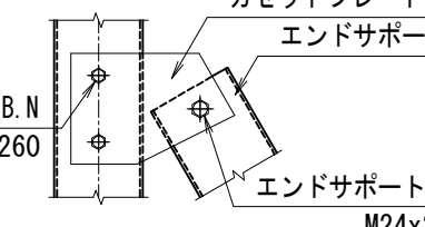
端柱・ワイヤー取付詳細
