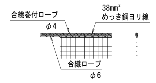
ネット取付詳細
