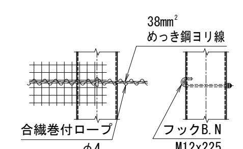
主柱・中間ワイヤー取付詳細
