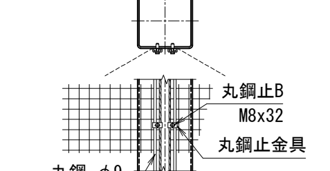
隅柱・ネット取付詳細
