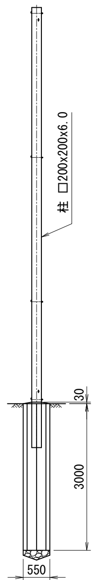
側面図 (S=1/80)
