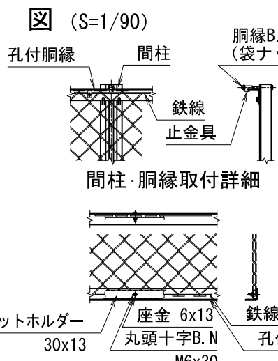
ネットホルダー取付詳細
