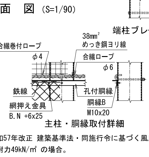
主柱・胴縁取付詳細
