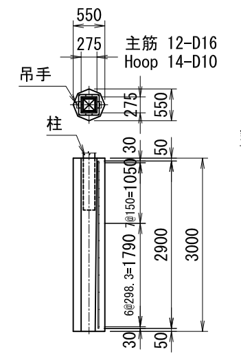
P型基礎コンクリート配筋図
