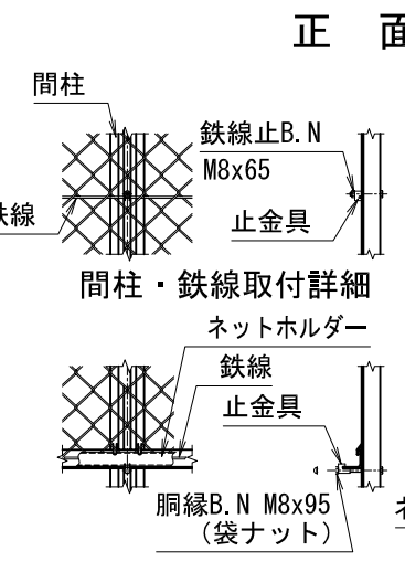
下胴縁取付詳細
