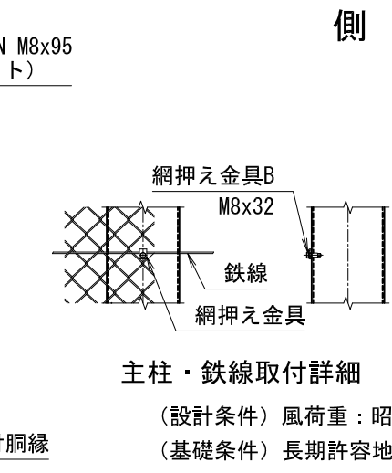
主柱・鉄線取付詳細
