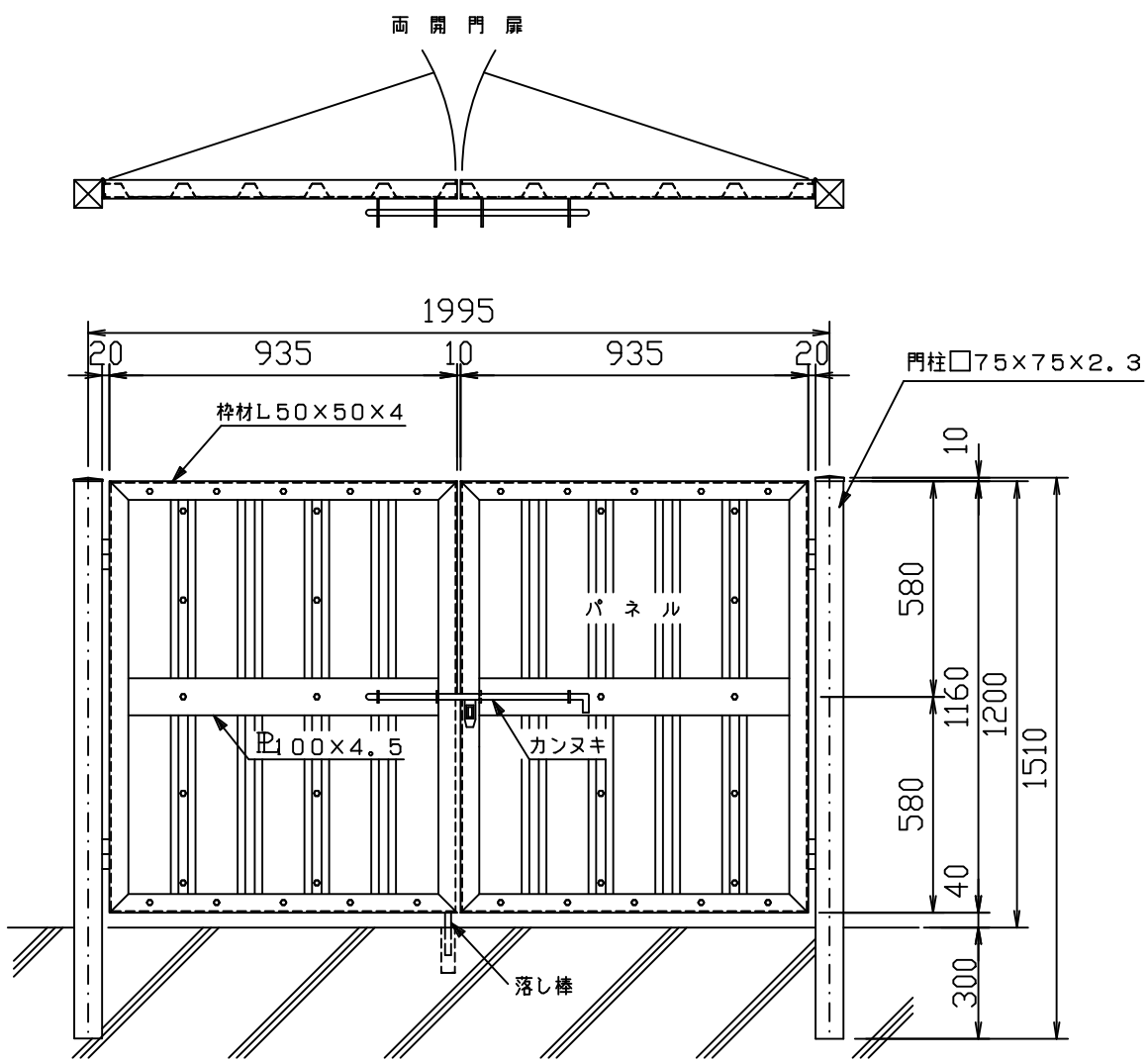
正面図 (S=1/15)
