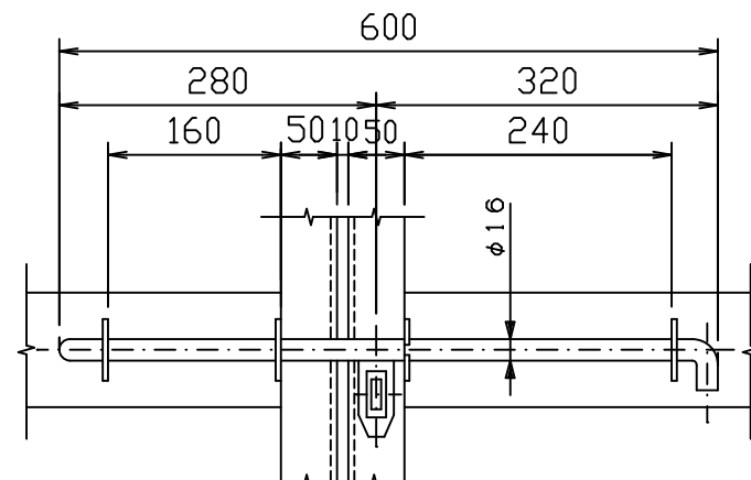
両開カンヌキ詳細
