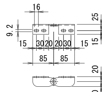
自在胴縁継手
