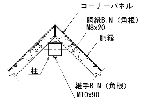
出隅取付詳細
