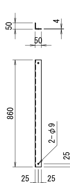
額縁詳細図
