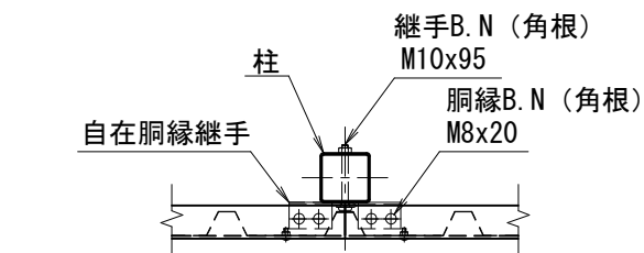
柱・胴縁取付詳細
