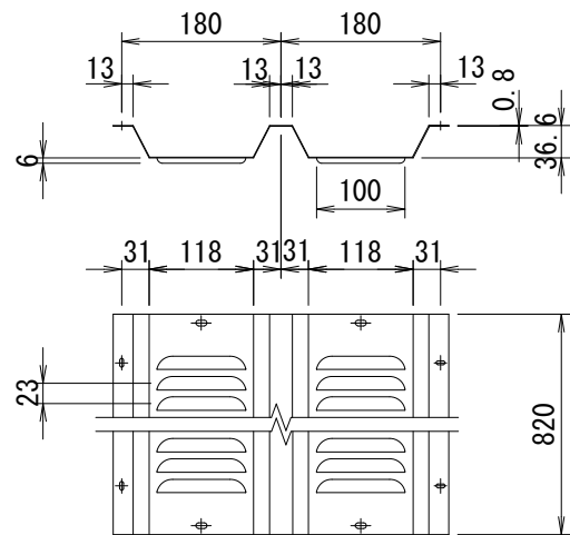
正面図 (S=1/20)
