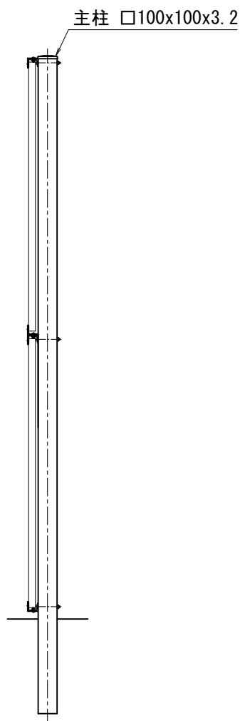
側面図 (S=1/30)
