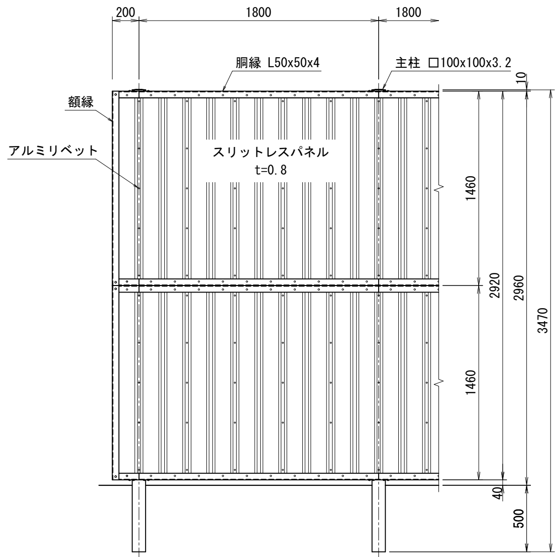
正面図 (S=1/30)
