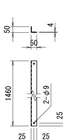
額縁詳細図
