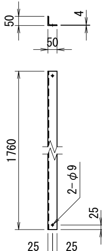
額縁詳細図
