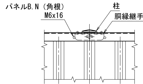
柱・胴縁取付詳細
