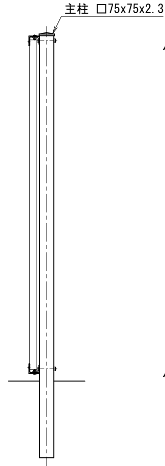
側面図 (S=1/20)
