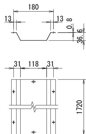
調整パネル詳細図
