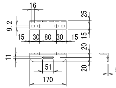
胴縁継手
