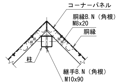
出隅取付詳細
