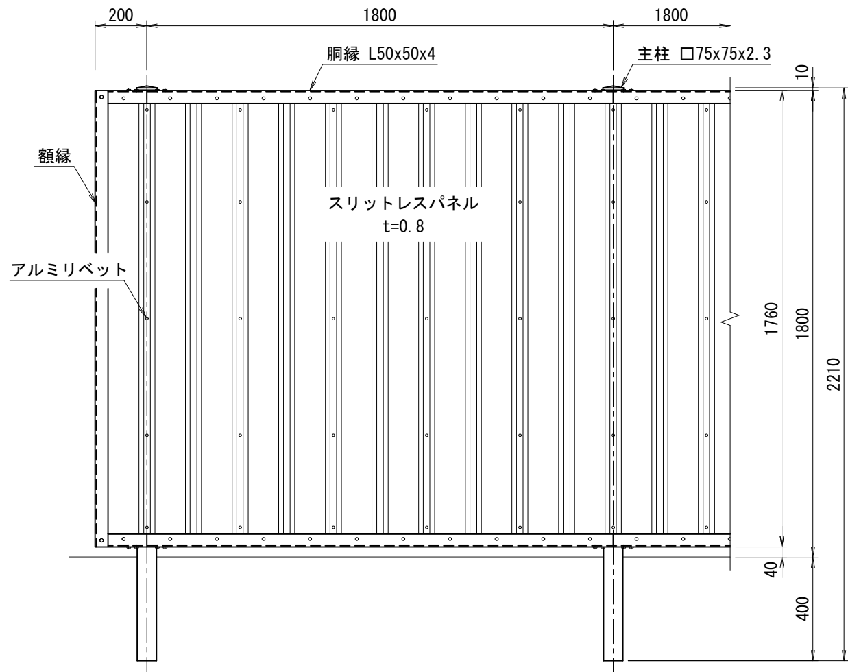
正面図 (S=1/20)
