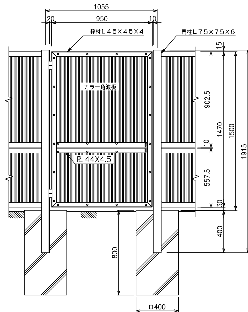
正面図 (S=1/15)
