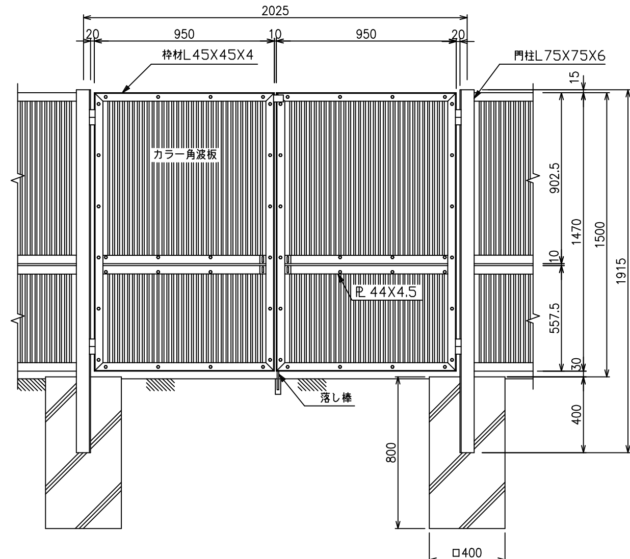
正面図 (S=1/15)
