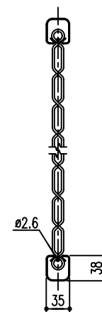
胴縁と金網取付断面図
