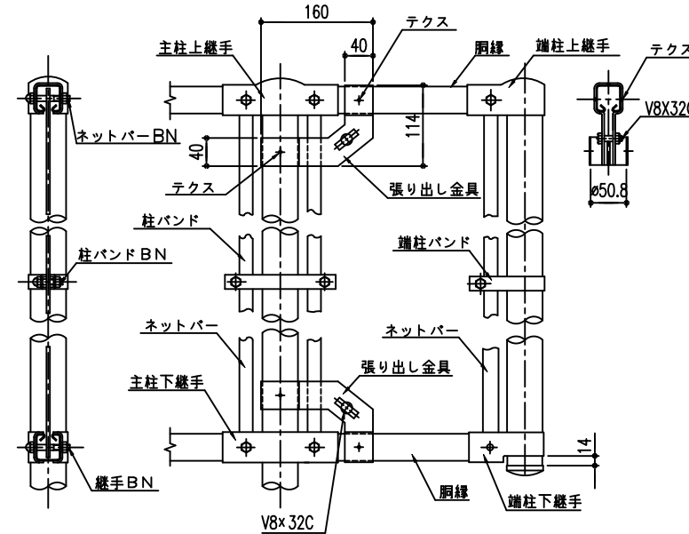
支柱・張り出し部取付詳細 S=1/6
