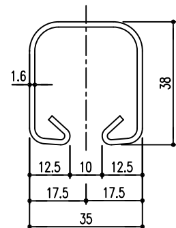
胴縁断面図 S=1/1
